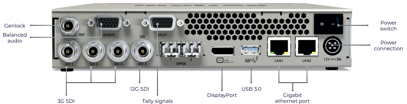
Matrox Monarch EDGE D4 (back view)
